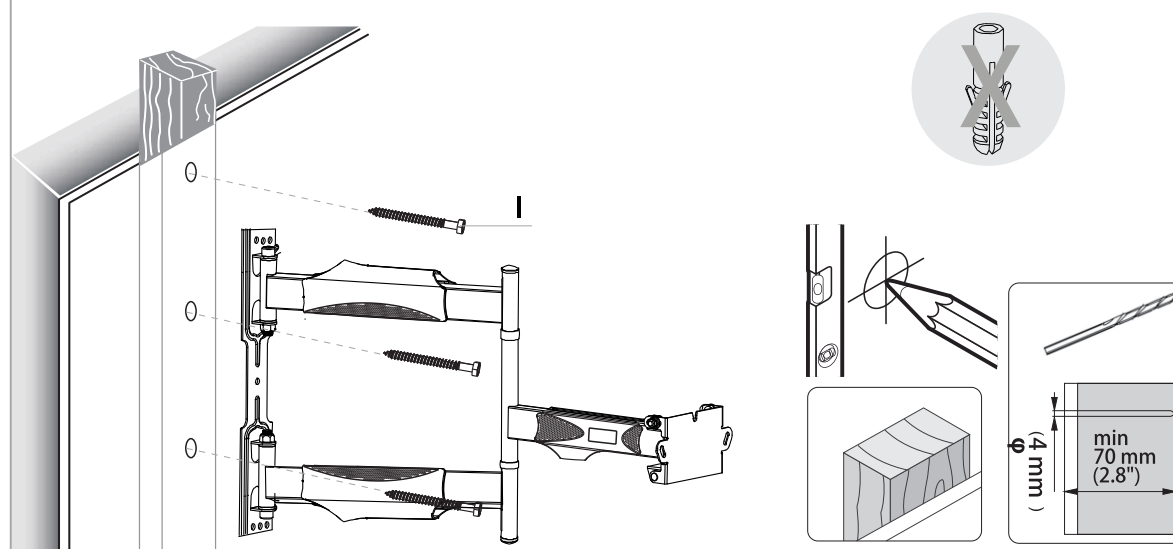
4. שחרור בורג
